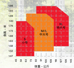
保泰特P200全身式安全带尺码表
